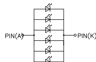
背光电路图 (CIRCUIT DIAGRAM)
